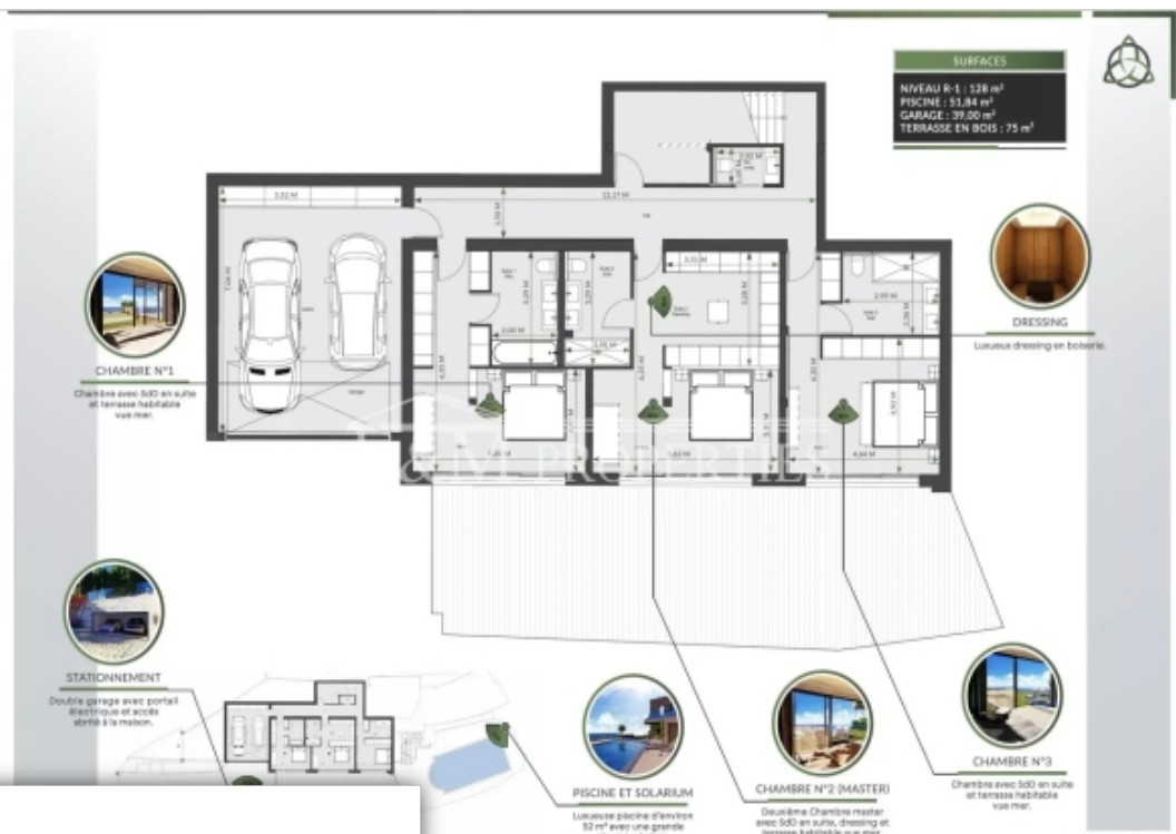
PLAN NIVEAU R-1
